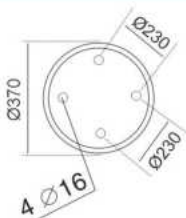
CHÂN ĐẾ 10 H1180 - Nhôm 13.300.000đ
