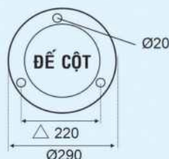
TRỤ 337 L660 x H4050 E27 x 2 14.500.000đ
