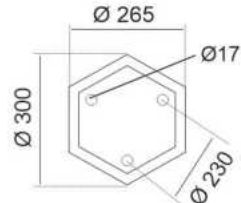
CHÂN ĐẾ 03 H630 - Nhôm 4.580.000đ
