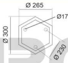
CHÂN ĐẾ 11 H630 - Nhôm 4.850.000đ
